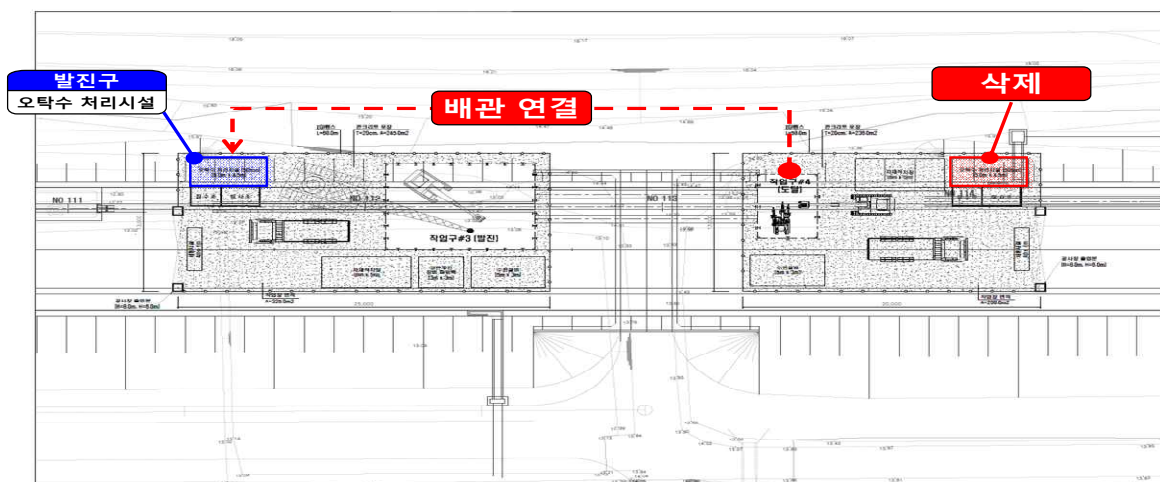
[그림 2] 오락수 처리시설 개선 사례(발진구1개소)
